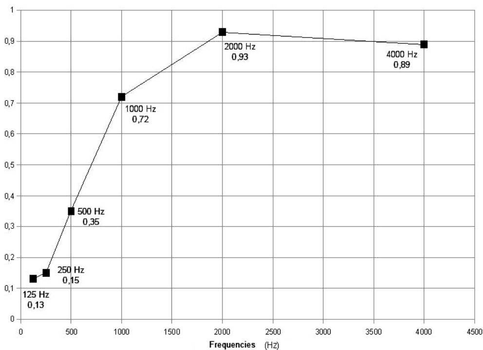
diagramme d'absorption en fonction de la fréquence
